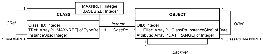
Fig. 1. OCB database schema
